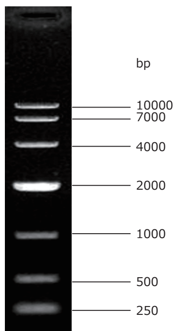
1% Agarose の電気泳動図
